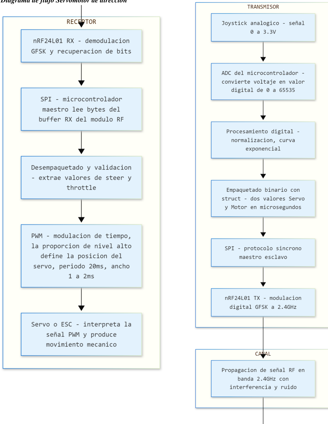
Diagrama de flujo Servomotor de dirección
