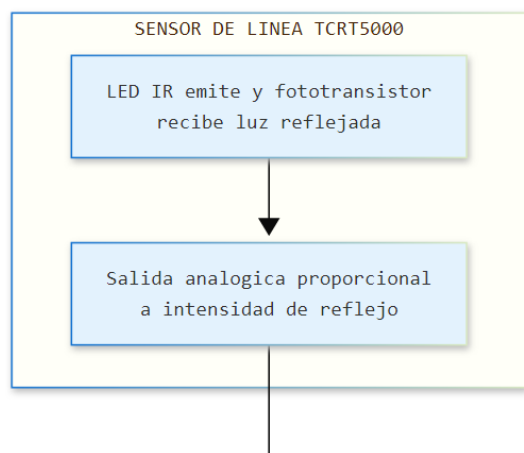
Diagrama de flujo Sensor de línea TCRT5000
