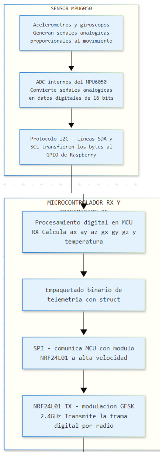
Diagrama de flujo sensor MPU6050
